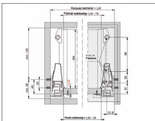
Szerelési méretek 164 mm magas fiókkoldal alkalmazása esetén
