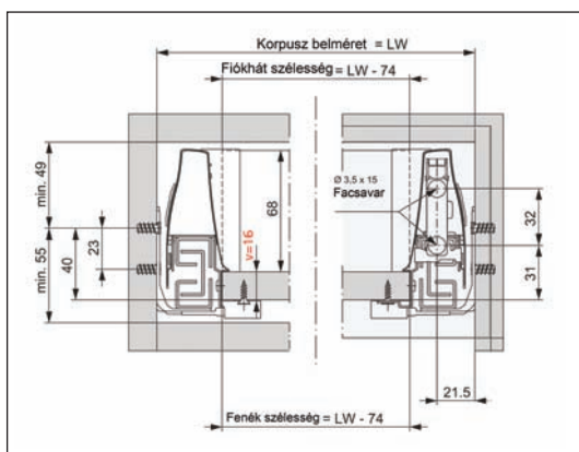
Szerelési méretek 86 mm magas fiókkoldal alkalmazása esetén
