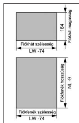
A fiókhát és fenék méretei v= 16 mm!
