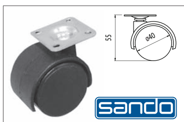
P-03 Talpas, \varnothing 40 mm Talpmagasság: 55 mm Talpméret: 35x35 mm Teherbírás: 20 kg szín: fekete 00002301000
