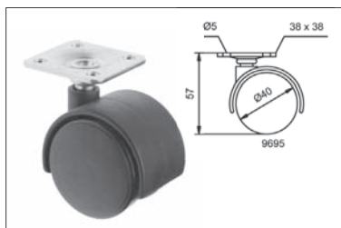
9695 Talpas, \varnothing 40 mm Talpmagasság: 57 mm Teherbírás: 30 kg szín: fekete 00002300600
