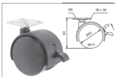
9613 Fékezős, talpas, \varnothing 50 mm Talpmagasság: 68 mm Teherbírás: 40 kg szín: fekete 00002300500
