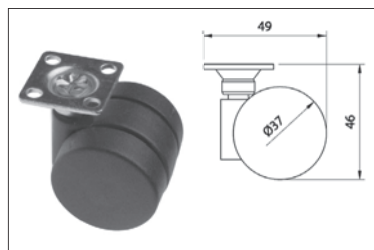
RA 037 Talpas, \varnothing 37 mm Talpméret: 28x28 mm Talpmagasság: 46 mm Teherbírás: 25 kg fekete 00002302000 aluminium 00002302010
