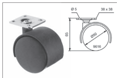
9616 Talpas, \varnothing 50 mm Talpmagasság: 65 mm Teherbírás: 40 kg szín: fekete 00002300700
