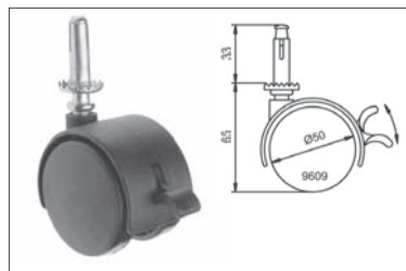
9609 Fékezős, hüvelyes, \varnothing 50 mm Talpmagasság: 65 mm Hüvely: \varnothing 9,5 mm Teherbírás: 40 kg szín: fekete 00002300400
