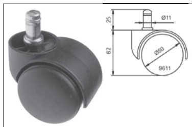
9611 Csapos, \varnothing 50 mm Talpmagasság: 62 mm Teherbírás: 40 kg szín: fekete 00002300300
