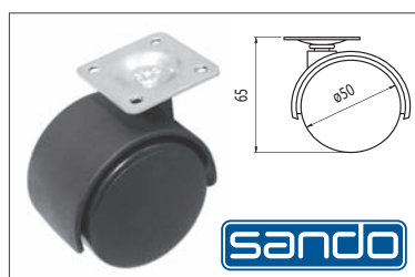
P-04 Talpas, \varnothing 50 mm Talpmagasság: 65 mm Talpméret: 38x38 mm Teherbírás: 25 kg szín: fekete 00002301100
