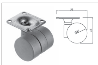
RA 137 Talpas, \varnothing 37 mm Talpmagasság: 46 mm Teherbírás: 50 kg fekete 00002302100 aluminium 00002302110
