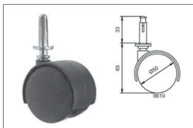
9610 Hüvelyes, \varnothing 50 mm Talpmagasság: 65 mm Hüvely: \varnothing 9,5 mm Teherbírás: 40 kg szín: fekete 00002300200
