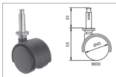
9600 Hüvelyes, \varnothing 40 mm Talpmagasság: 55 mm Hüvely: \varnothing 9,5 mm Teherbírás: 30 kg szín: fekete 00002300100
