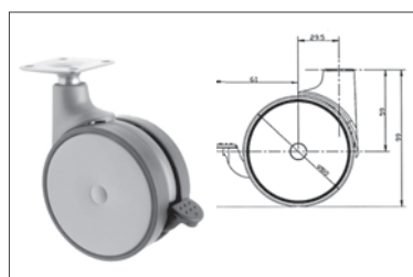
SLIM 80 Talpas, \varnothing 80 mm Talpméret: 42x42 mm Talpmagasság: 110 mm Teherbírás: 80 kg szín: alumínium fékezős 00002302210 fék nélkül 00002302200
